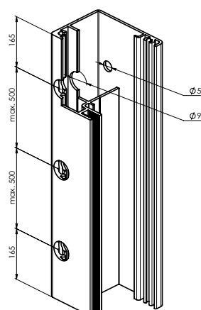
A840-1c vrtání čelně
